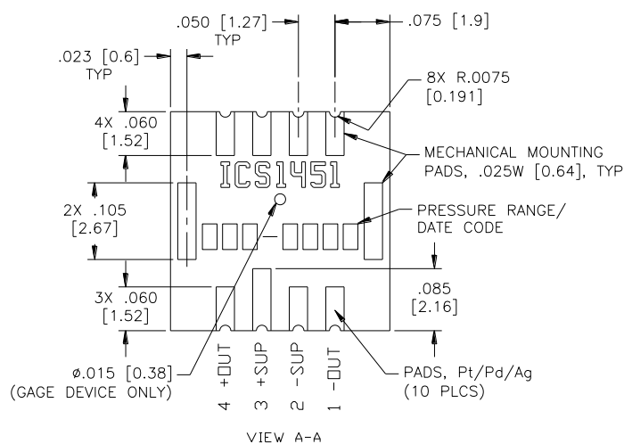
VIEW A-A
